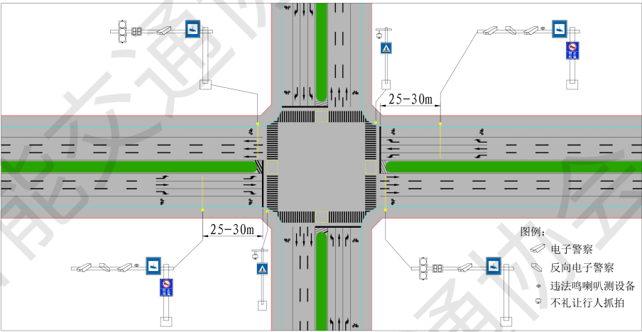
图 A.1 道路交通违法监测设施布设示意图
