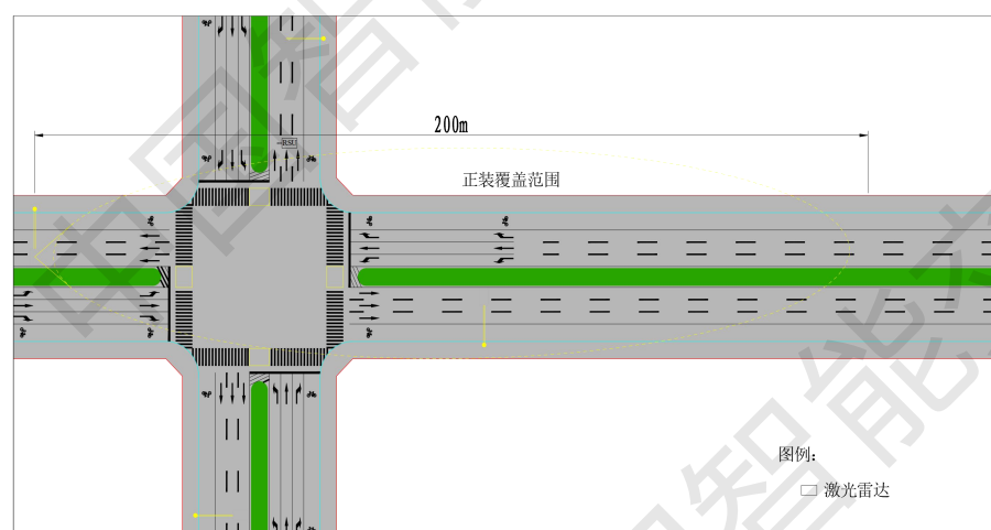
图 A. 5 激光雷达正装示意图
