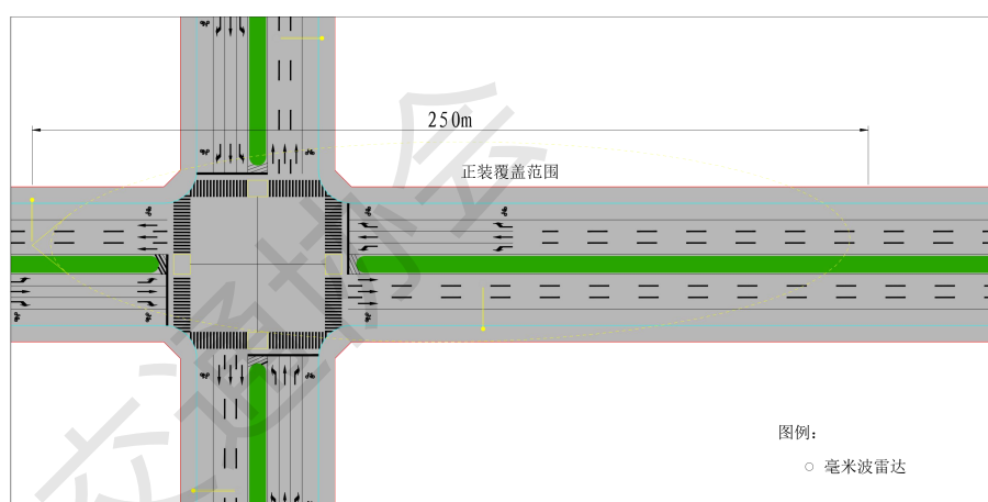
图 A. 3 毫米波雷达正装示意图
