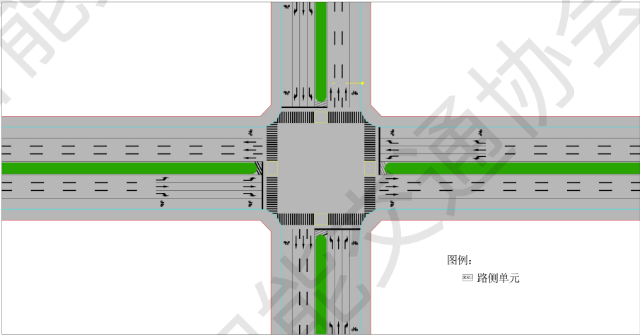
图 A.7 路侧单元布设示意图
