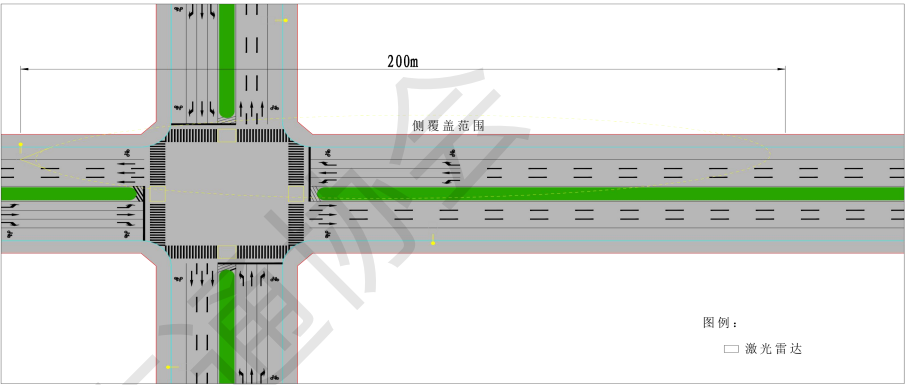
图 A.6 激光雷达侧装示意图
